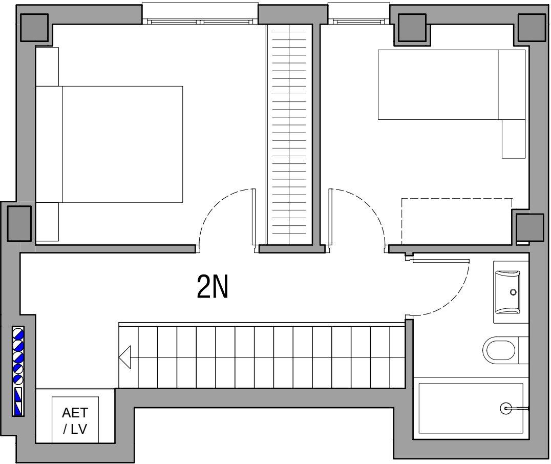
PLANTA PRIMERA
